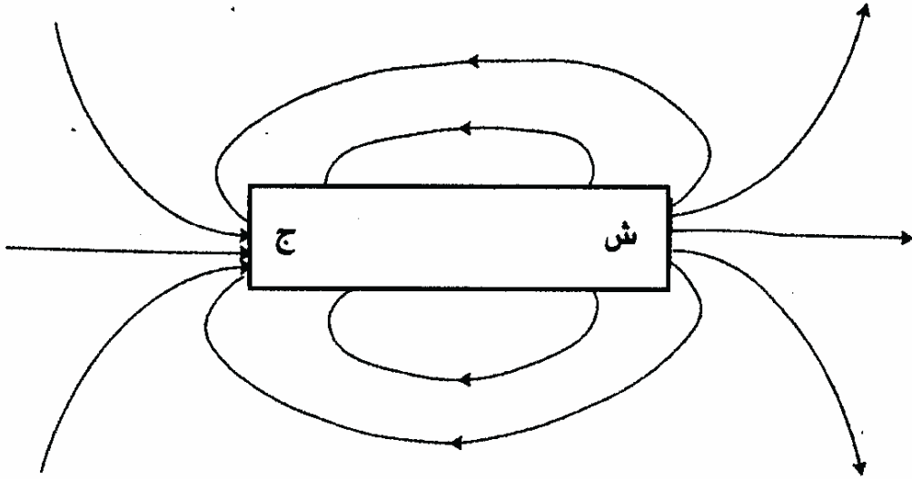
(الشكل 37): مغناطيس ثنائي القطب بحقل مغناطيسي جنوبي وشمالي. تتجه خطوط الحقل من الشمال إلى الجنوب.
